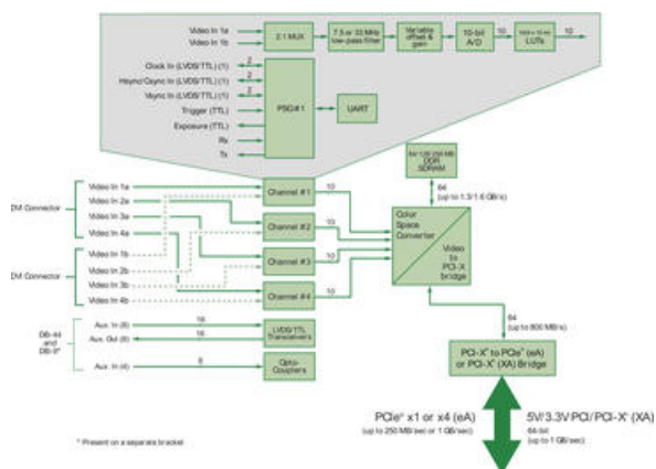
Blockdiagram för Matrox Solios eA/XA
