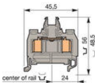
Standard 5 mm plint. Bredd 5 mm.
