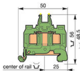
Plint för jordkabel. Bredd 6 mm.
