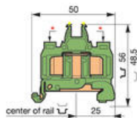
Plint för jordkabel. Bredd 8 mm.
